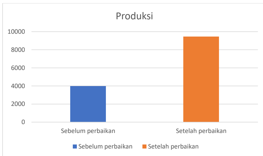
Gambar 4. Produktivitas Teoritis Alat Angkut Hino 500 Sebelum dan Setelah Perbaikan
