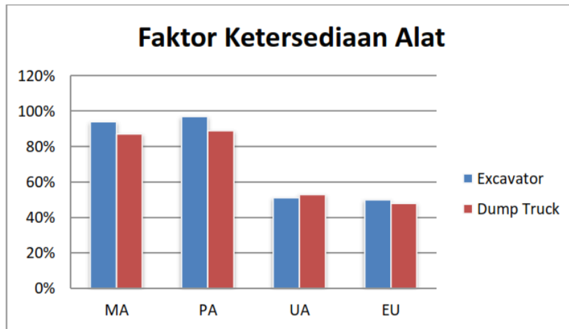
Gambar 2. Perbandingan Ketersediaan Alat Gali Muat Excavator PC 200 dan Alat Angkut Hino 500
