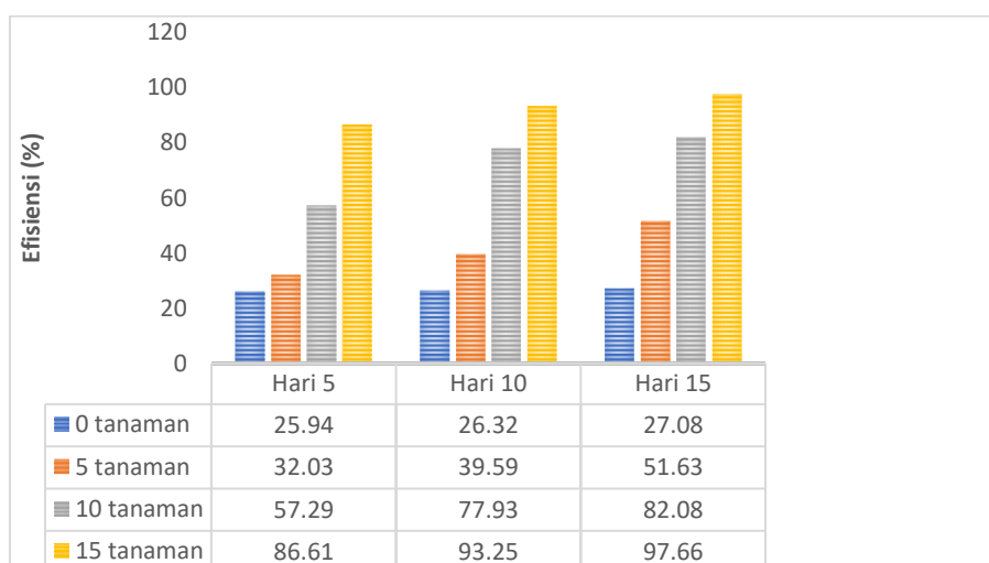
Gambar 4. Efisiensi Penurunan BOD dengan variasi waktu kontak dan jumlah tanaman
