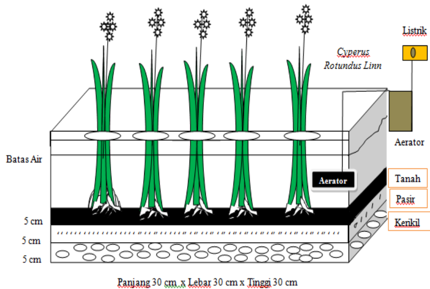
Gambar 1 Desain proses Fitoremediasi
