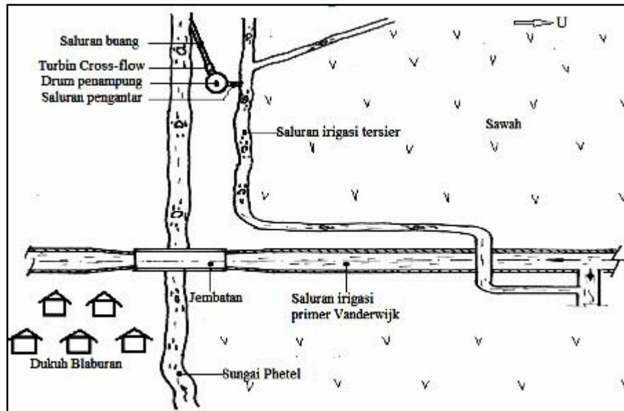
Gambar 1. Lay-out di Sekitar Lokasi PTMPMD, Dukuh Blaburan, Desa Bligo, Kecamatan Ngluwar, Kabupaten Magelang
