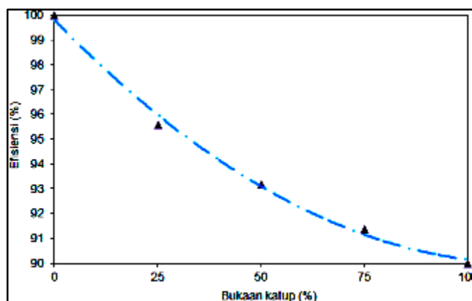
Gambar 11. Trend Efisiensi Regulator-Katup
