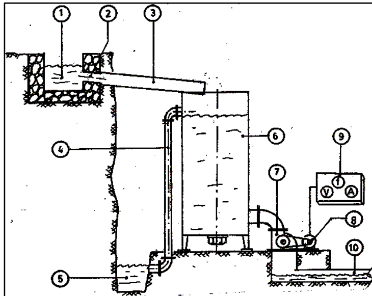
Gambar 6. Sistem PTMPMD
