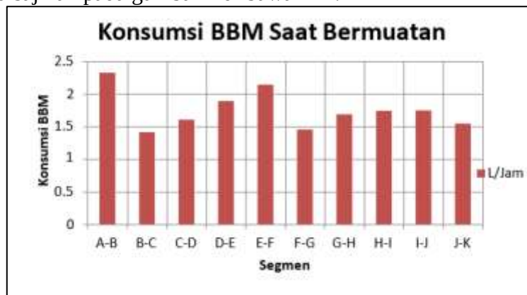
Gambar 2. Konsumsi bahan bakar saat bermuatan
