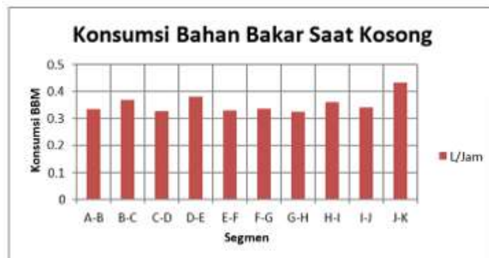
Gambar 4. Konsumsi bahan bakar saat kosong
