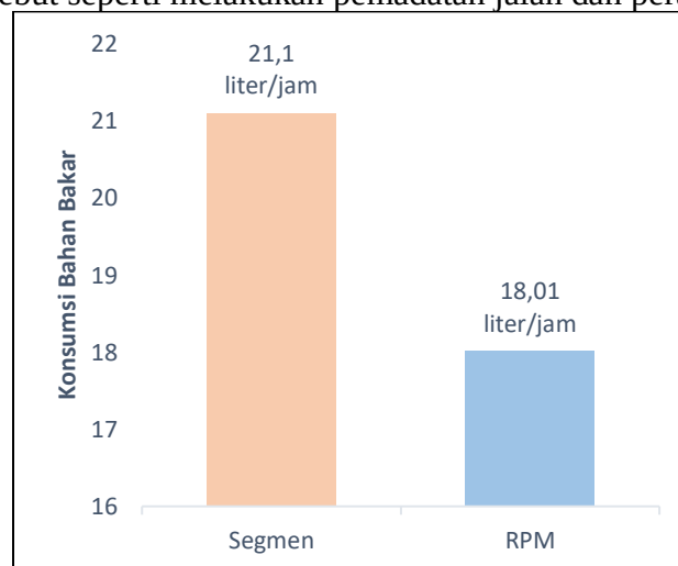
Gambar 4. Perbandingan konsumsi bahan bakar
