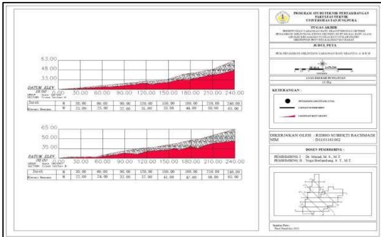
Gambar 6. Peta Penampang Melintang Cadangan Batu Granit A'-A' dan B'-B'
