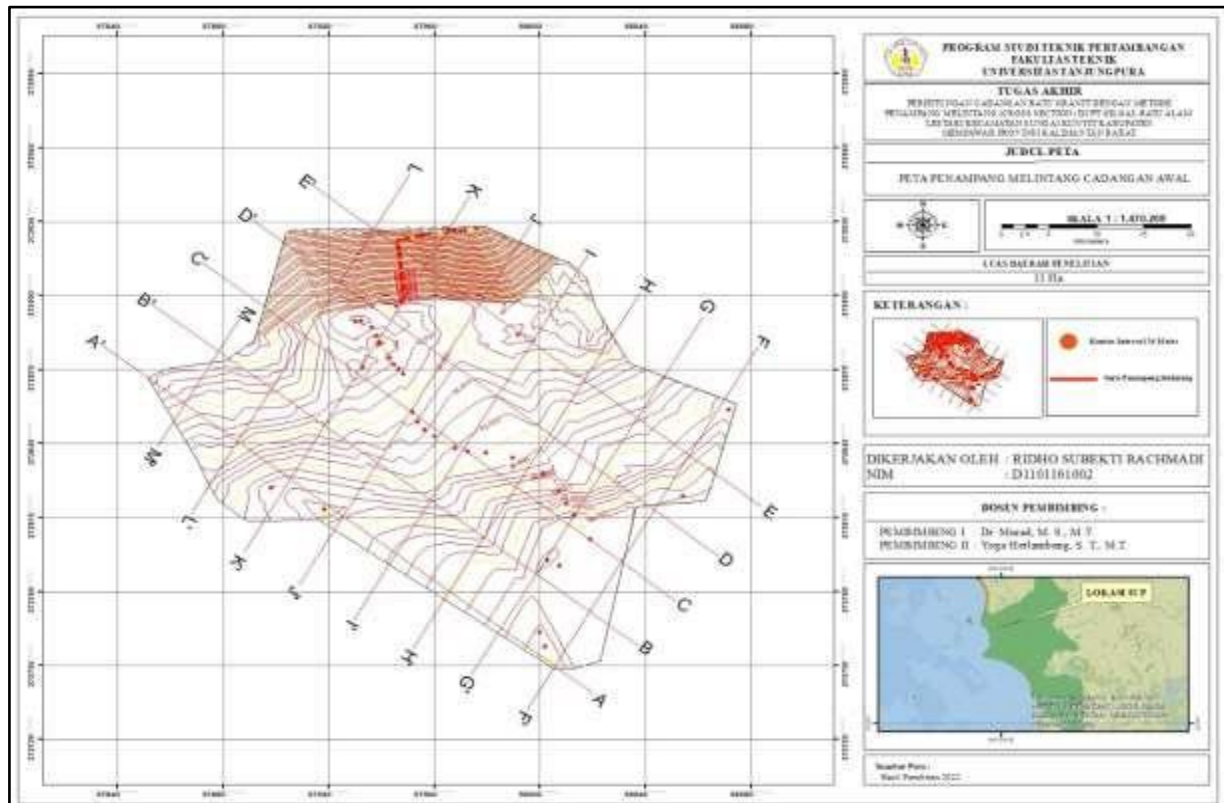
Gambar 4. Peta Penampang Melintang Cadangan Awal
