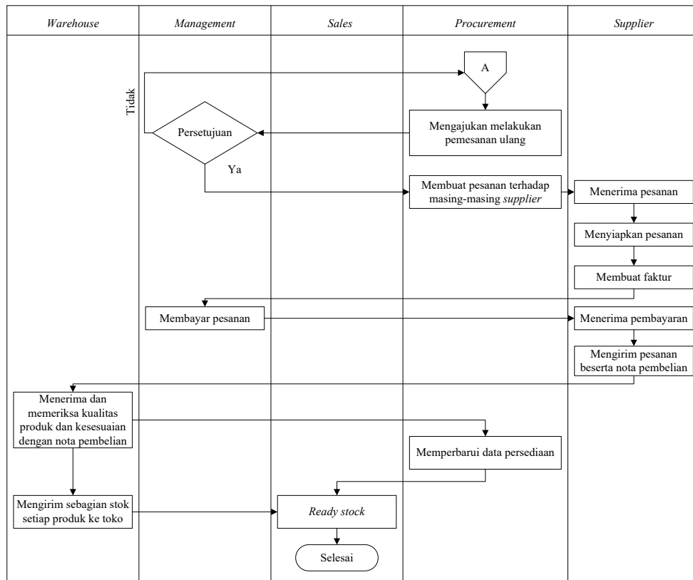
Gambar 5. Flowchart sistem pengendalian persediaan baru produk dental (lanjutan)
