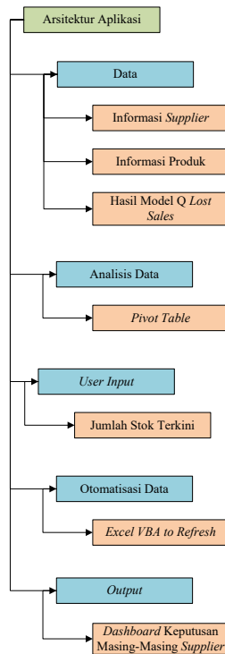
Gambar 6. Arsitektur aplikasi
