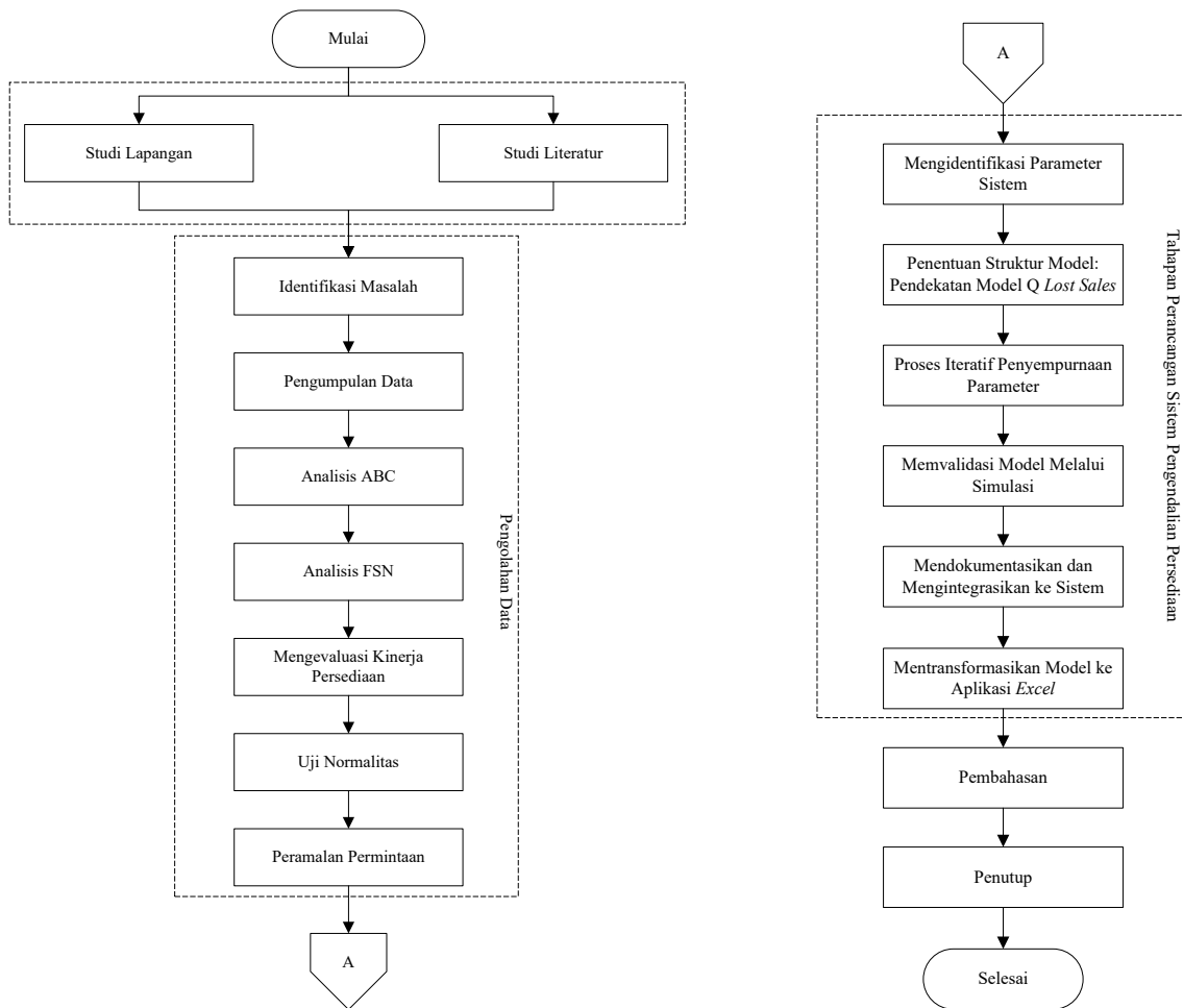
Gambar 2. Tahapan penelitian
