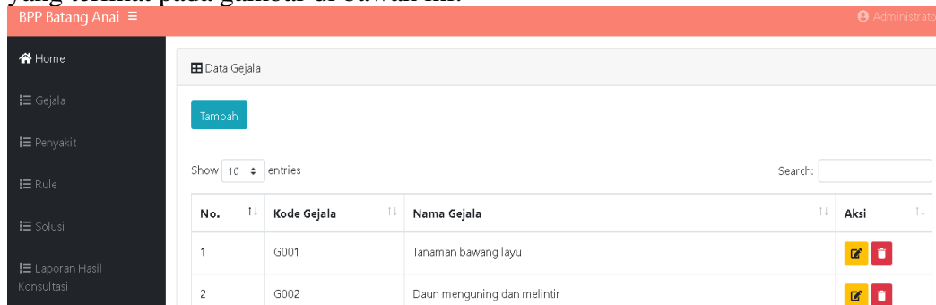
Gambar.8 Menu Gejala
