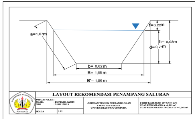
Gambar 2. Dimensi penampang
